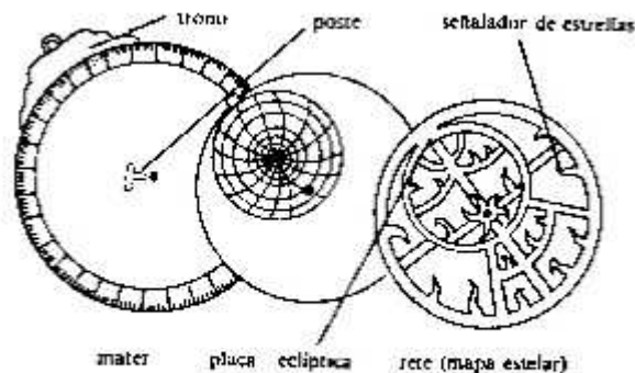
Los componentes de un astrolabio plano.
